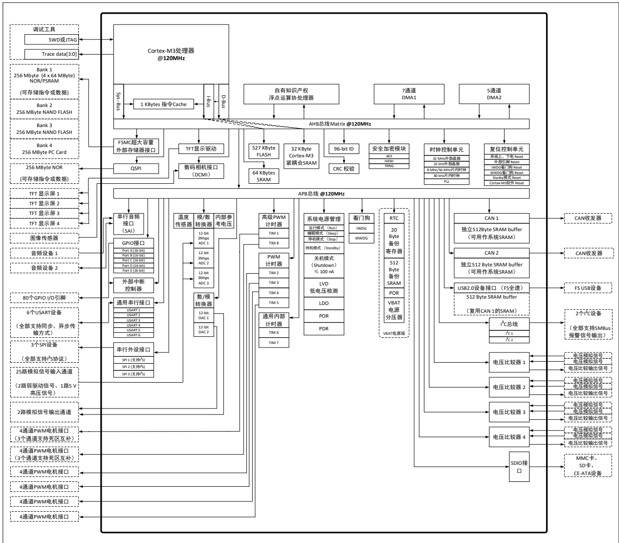
图 3-1 HK32F39A MCU 的功能框图
