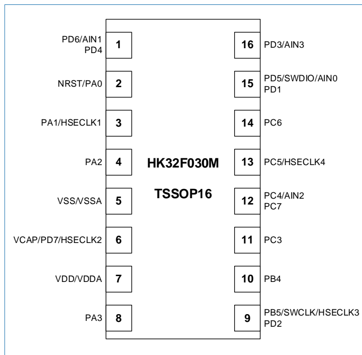
图 6-2 TTSOP16 (HK32F030MD4P6) 封装
