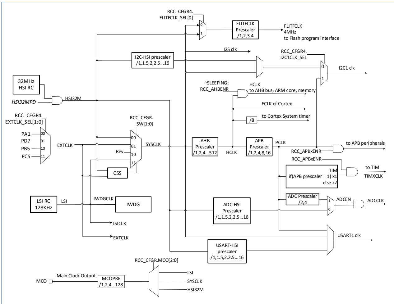
图 3-4 时钟树
